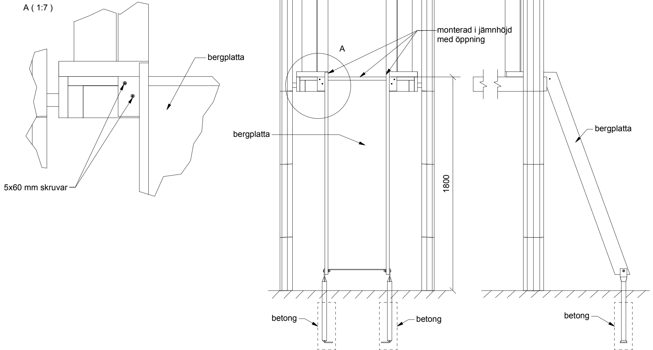
66: Detalj bergplatta på Robinia tårn
